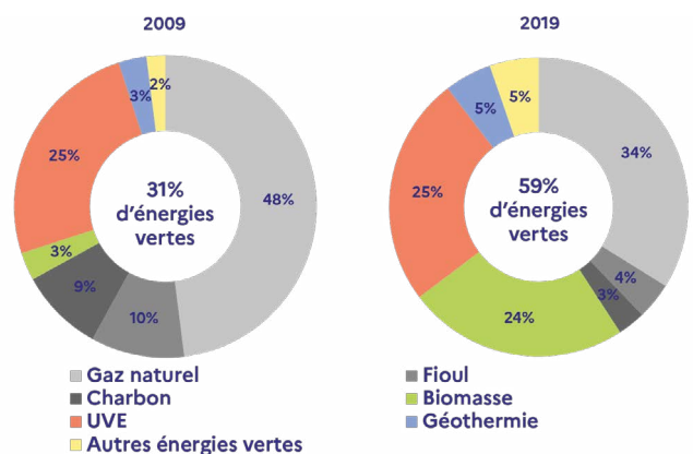
Évolution du bouquet énergétique des réseaux de chaleur entre 2009 et 2019
